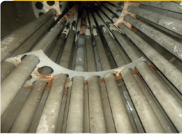
CAMBIOS DE 2 BAFLES Y REPOSICIÓN DE 20 TUBOS EN SECADOR BM-513
