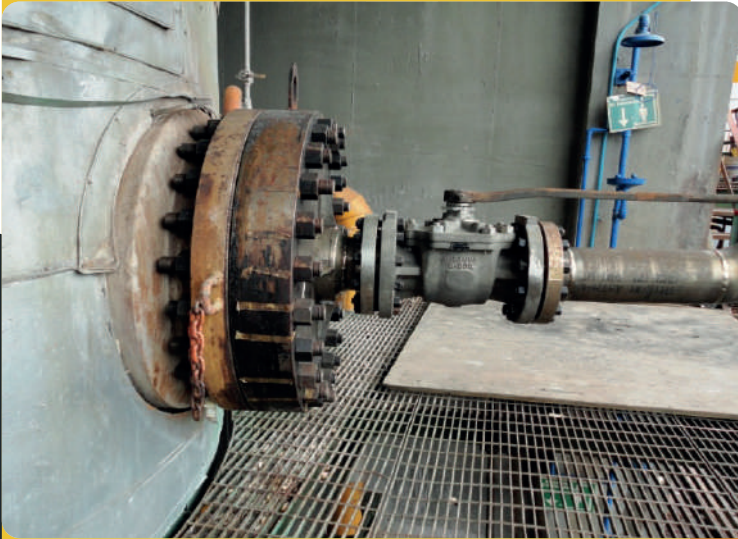
INSTALACIÓN DE LINEA DE REFLUJO A LOS REACTORES BR-305 Y BR-307
